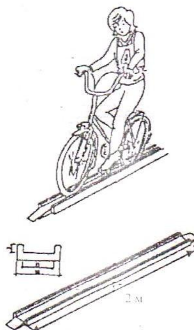
Рис. 2. Рельсы «Желоб»
